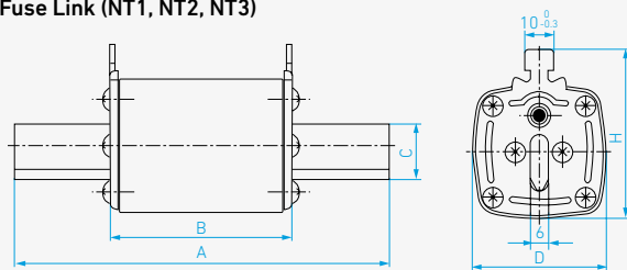
Fuse Link (NT1, NT2, NT3)
