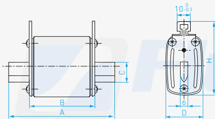
Fuse Link (NT00, NT0)
