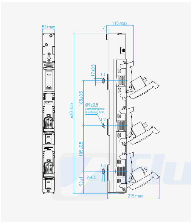
HC-U / 160 AF
