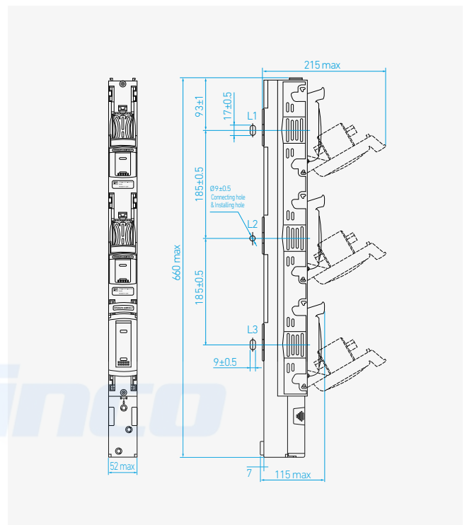
HC-D / 160 AF
