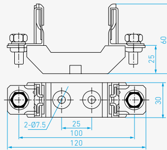
Fuse Base (NT00)
